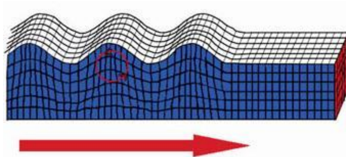
Ondas Rayleigh www.funvisis.gob.ve
