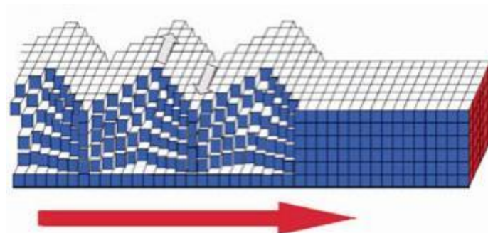
Ondas Love www.funvisis.gob.ve
