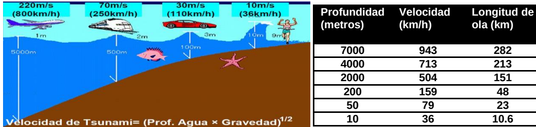
Velocidad de propagación de tsunamis en función de la profundidad
