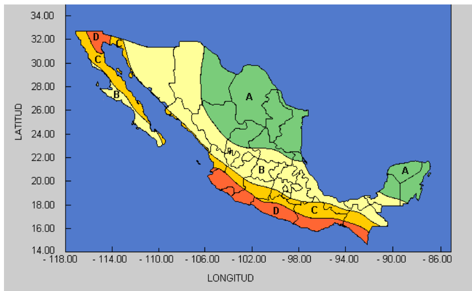
Regionalización sísmica de la República Mexicana
