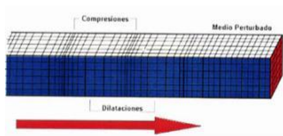
Ondas P
