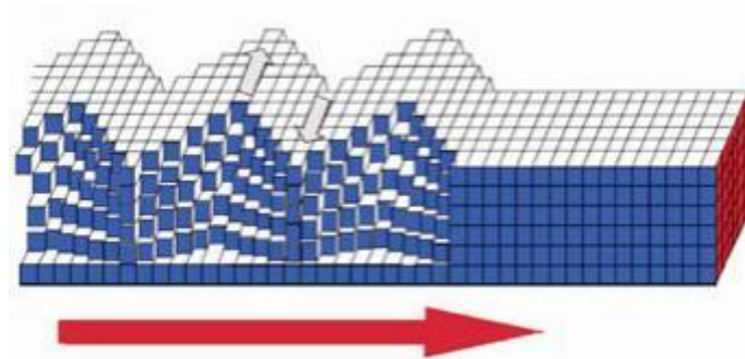
Ondas Love
