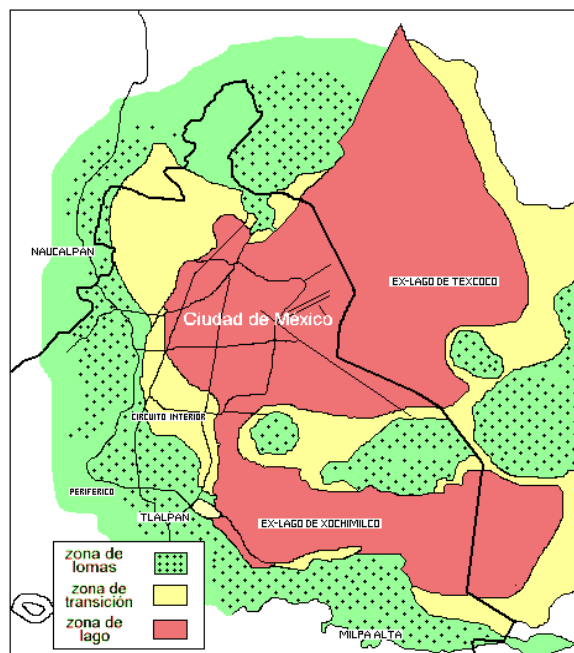
Zonificación estratigráfica de la Ciudad de México
