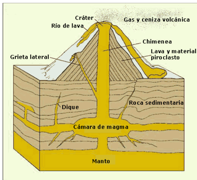
Figura 4.- http://centros3.pntic.mec.es/cp.valvanera/volcanes/partes/partes.html
