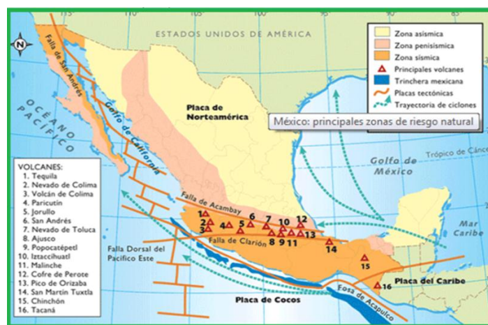
Figura 1. http://mx.kalipedia.com/geografia-mexico/tema/mexico/zonas-volcanicas.html
